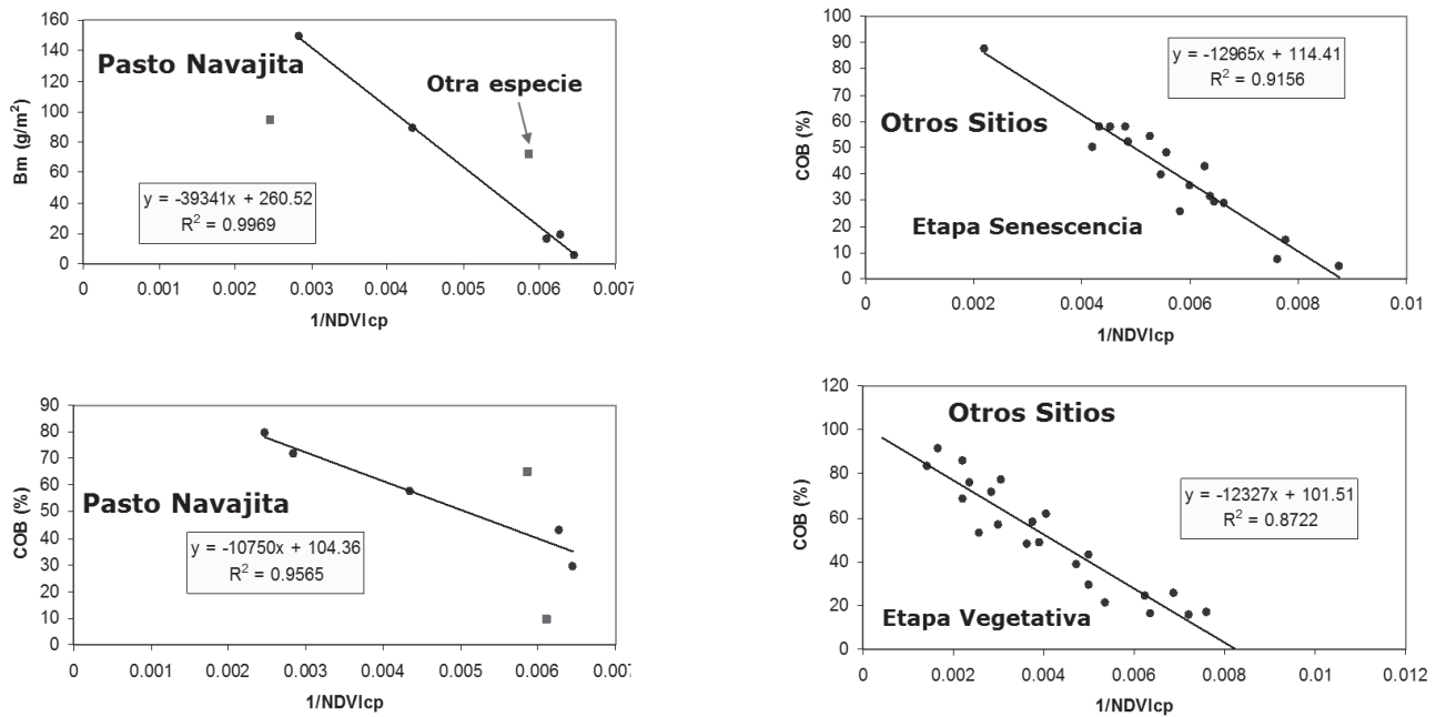
Figura 9. Relación (1/NDVI cp )-Bm y COB para un sitio de control (pasto navajita; Bouteloa spp. ) y (1/NDVI cp )-COB para sitios no control, etapa vegetativa y de senescencia. Bm = biomasa; COB = cobertura aérea.
