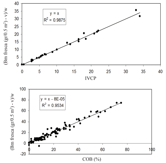
Figura 11. Relaciones estandarizadas ente el IVCP y la Bm fresca y la COB y la Bm fresca de diferentes sitios de muestreo de la campaña del 2007. Bm = biomasa; COB = cobertura aérea.
