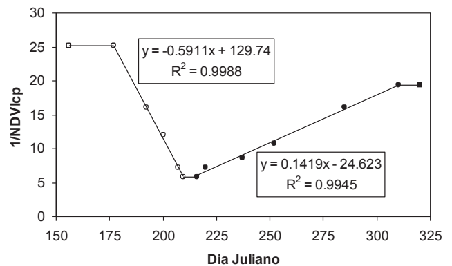
Figura 2. Patrones temporales de 1/NDVIcp para un pasto. Los puntos cuadrados fueron puestos en forma artificial para las mesetas.
