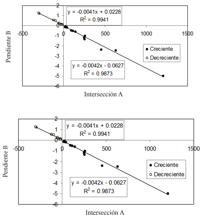
Figura 13. Patrones entre los parámetros de la evolución temporal de la biomasa evaluada en campo, para la etapa vegetativa (creciente) y de senescencia (decreciente).
