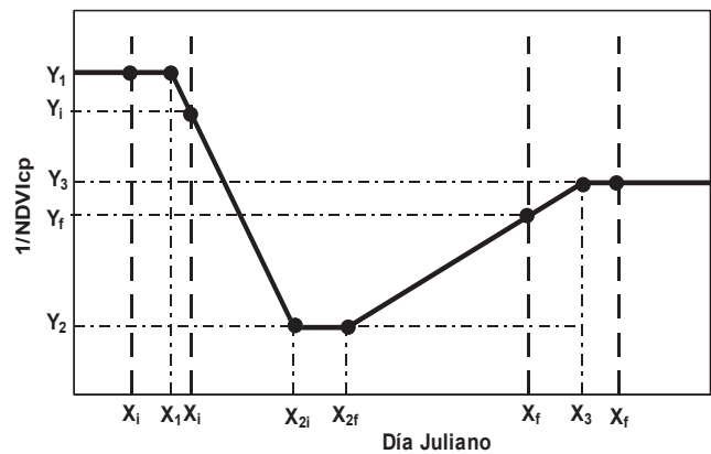
Figura 3. Modelo propuesto para la evolución temporal de 1/NDVIcp.
