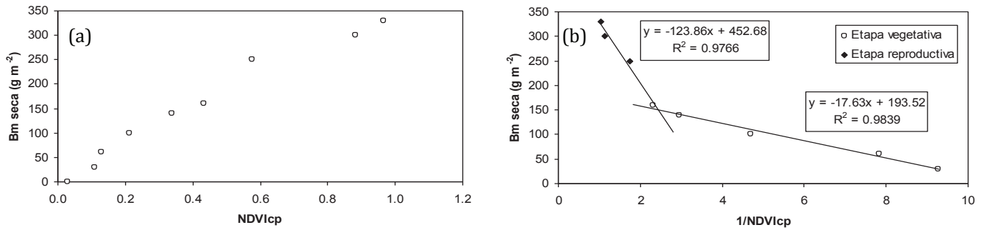
Figura 1. (a) Relación entre la Bm (biomasa) seca y el NDVIcp y (b) relación entre la Bm seca y 1/NDVIcp.
