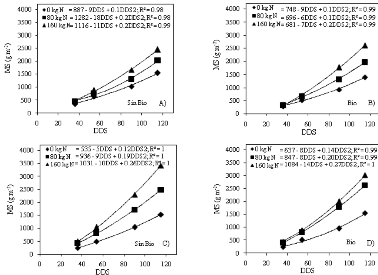
Figura 3. Dinámica de la materia seca total en maíz Vandeño (A y B) y H-562 (C y D) en función del nitrógeno y biofertilizante (Bio) (B y D) durante el ciclo del cultivo. Iguala, Gro. 2011.
