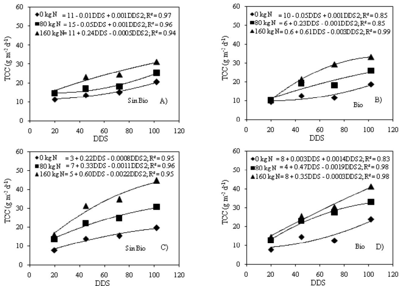
Figura 4. Dinámica de la tasa media de crecimiento del cultivo ( \overline{TCC} ) en maíz Vandeano (A y B) y H-562 (C y D) en función del nitrógeno y biofertilizante (Bio) (B y D). Iguala, Gro. 2011.
