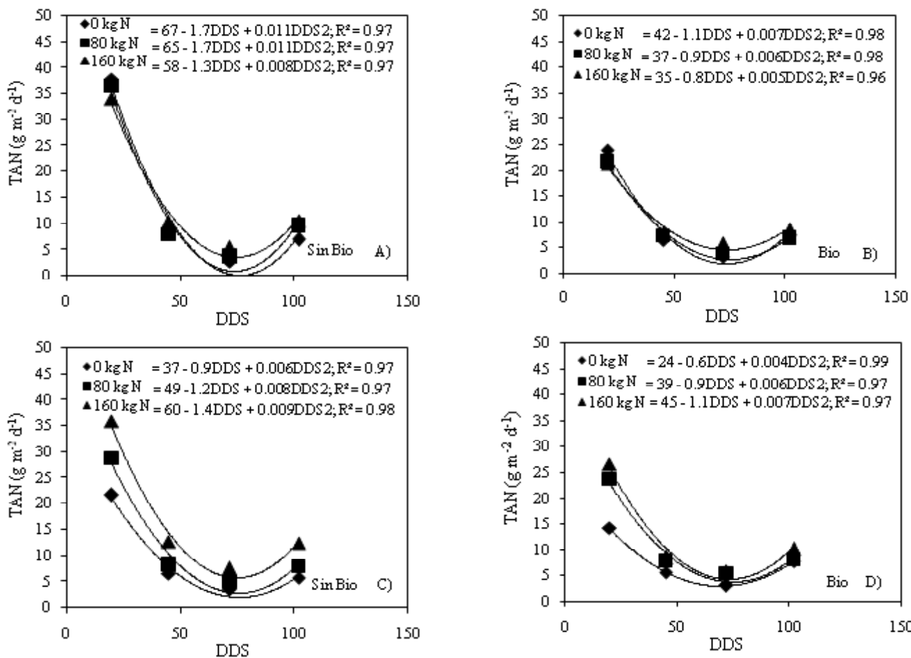
Figura 5. Dinámica de la tasa media de asimilación neta ( \overline{\text{TAN}} ) en maíz Vandeño (A y B) y H-562 (C y D) en función del nitrógeno y biofertilizante (Bio) (B y D). Iguala, Gro. 2011.
