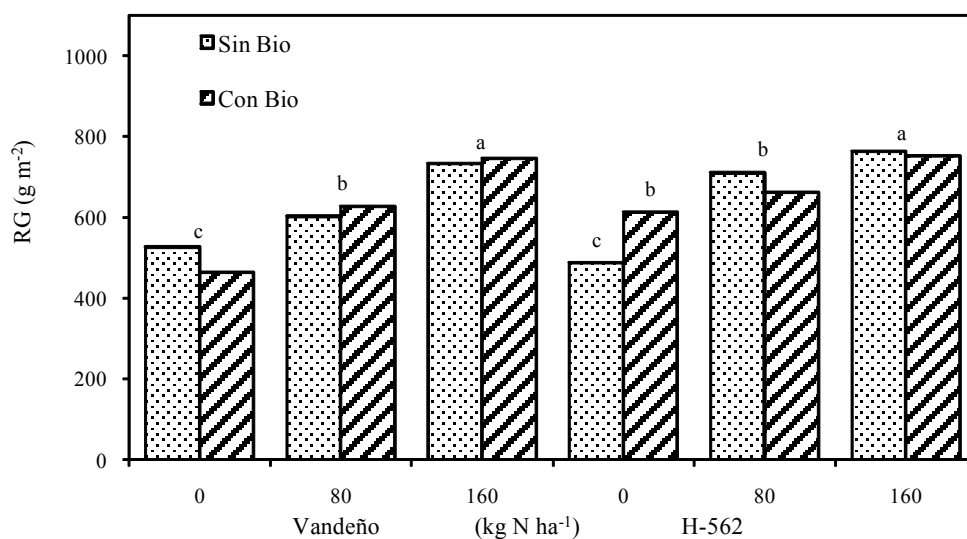
Figura 6. Rendimiento de grano (RG) en genotipos de maíz en función del biofertilizante (Bio) y nitrógeno (N). Iguala, Gro. 2011.
