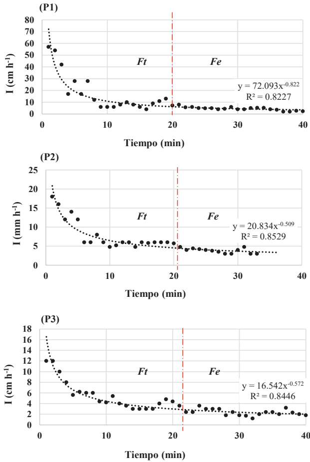
Figura 3. Comportamiento gráfico promedio del movimiento del agua a través del perfil a 30 cm de profundidad en los tres sitios de prueba (parcelas: P1, P2 y P3). Figure 3. Average graphical behavior of water movement through the profile at 30 cm depth at the three test sites (plots: P1, P2 and P3).
